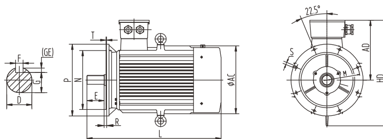
H315~355-IM V1
