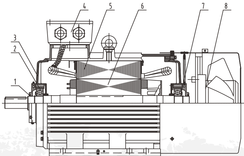
H80 ~ H355
